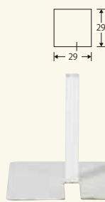
看板用ベース サイズ: W305×D365×H250 [コード] 15101-81
