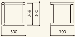
ステージシステム角トラス 30 サイズ:W300×D300×H300 [コード] 15053-03
