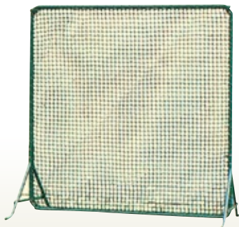
防球用ネットゲージ サイズ:W2,000×H2,000 [コード] 13003-84
