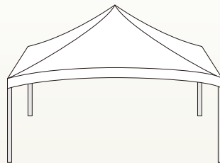
ビッグパワー-10・10 白 サイズ:W10,000×D10,000×H5,260 [コード] 15006-12
