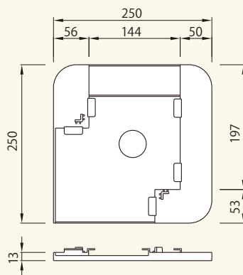
敷板 エコワイドベース角兼用 室内用 【コード】01075-03
