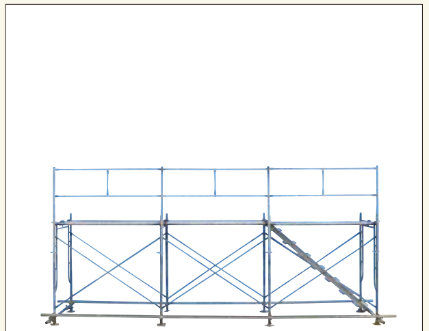
階段枠の取り付け
