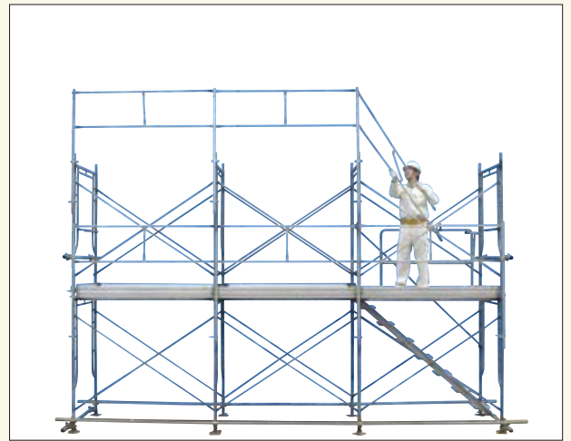
3段目の先行手摺の取り付け
