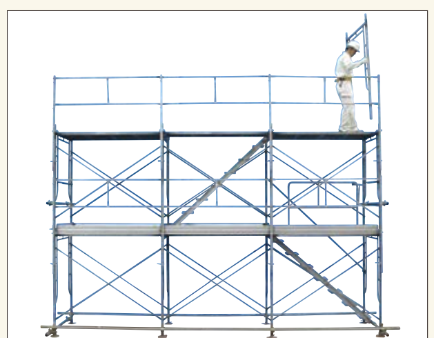
3段目の枠組の取り付け
