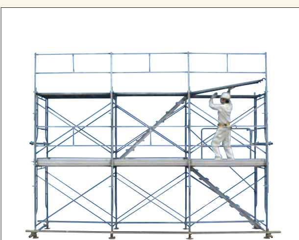
鋼製布板の取り付け 階段枠の取り付け
