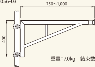
ブラケット NKB1000 [コード]01056-03
