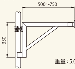
ブラケット NKB750 [コード]01056-02
