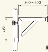
ブラケット NKB500 [コード]01056-01
